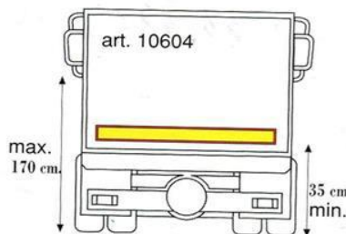
10604 Alluminio rifrangente/fluorescente mm. 1140x200 kit 1 pz.
