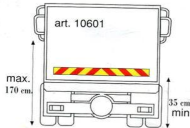
10601 Alluminio rifrangente/fluorescente mm. 1140x140 kit 1 pz.
