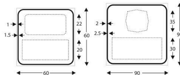
Segnali per Cavalcavia (Autostrade e strade statali)
